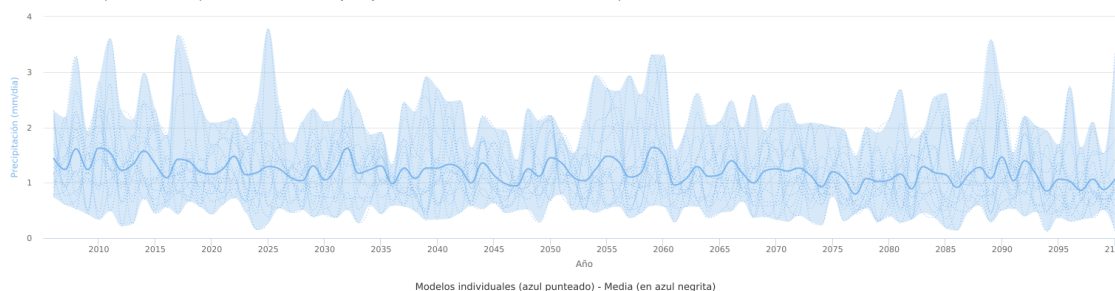
Escenarios AdapteCCa - Precipitación - Datos en rejilla ajustados (media) - RCP 8.5 - Año completo - Borriana/Burriana (Comunitat Valenciana)
