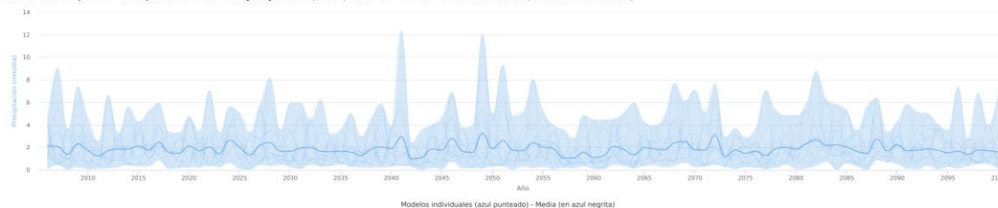
Escenarios AdapteCCa - Precipitación - Datos en rejilla ajustados (media) - RCP 4.5 - Otoño - Borriana/Burriana (Comunitat Valenciana)
