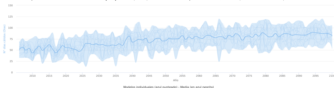
Escenarios AdapteCCa - N° días cálidos - Datos en rejilla ajustados (media) - RCP 4.5 - Año completo - Borriana/Burriana (Comunitat Valenciana)
