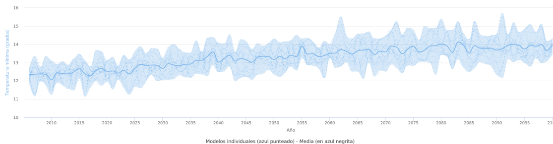
Escenarios AdapteCCa - Temperatura mínima - Datos en rejilla ajustados (media) - RCP 4.5 - Año completo - Borriana/Burriana (Comunitat Valenciana)
