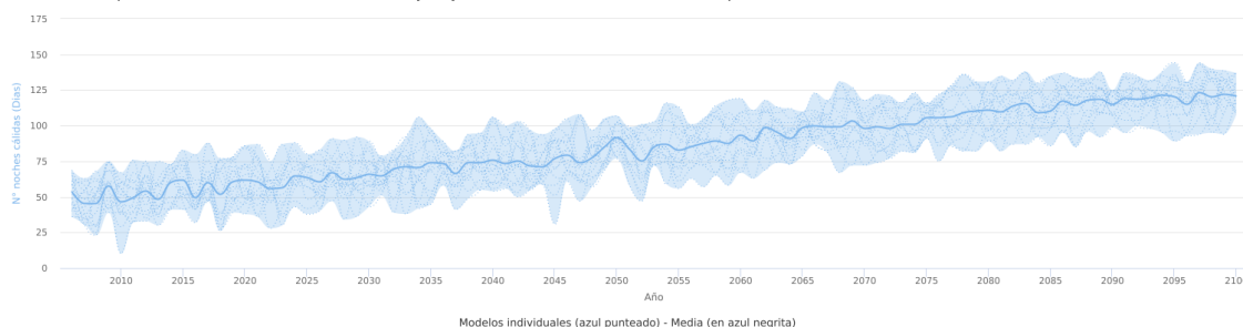
Escenarios AdapteCCa - N° noches cálidas - Datos en rejilla ajustados (media) - RCP 8.5 - Año completo - Borriana/Burriana (Comunitat Valenciana)
