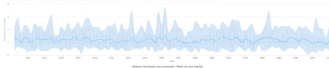
Escenarios AdapteCCa - Precipitación - Datos en rejilla ajustados (media) - RCP 4.5 - Año completo - Borriana/Burriana (Comunitat Valenciana)
