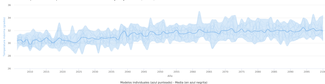
Escenarios AdapteCCa - Temperatura máxima - Datos en rejilla ajustados (media) - RCP 4.5 - Verano - Borriana/Burriana
