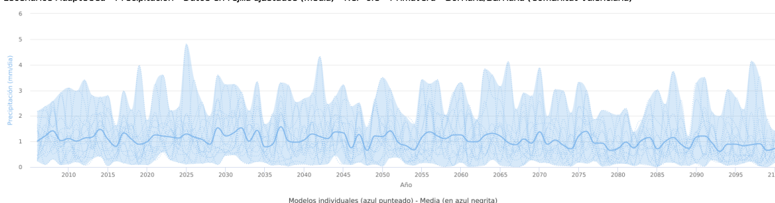
Escenarios AdapteCCa - Precipitación - Datos en rejilla ajustados (media) - RCP 8.5 - Primavera - Borriana/Burriana (Comunitat Valenciana)
