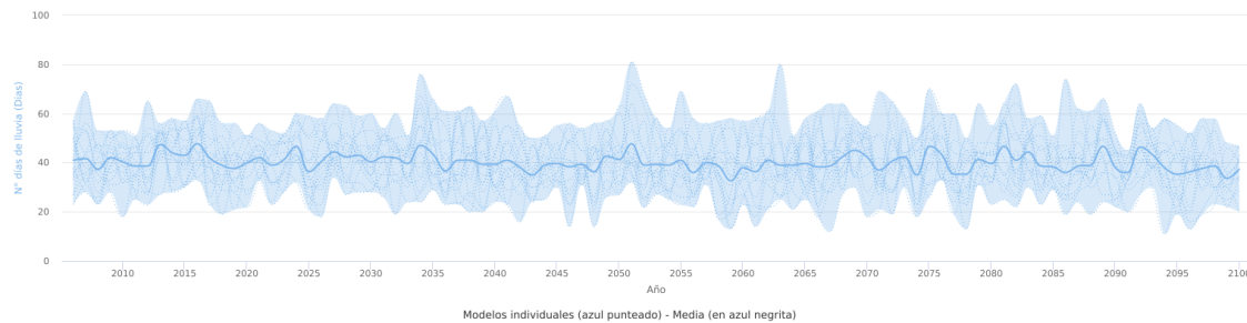
Escenarios AdapteCCa - N° días de lluvia - Datos en rejilla ajustados (media) - RCP 4.5 - Año completo - Burriana/Burriana (Comunitat Valenciana)
