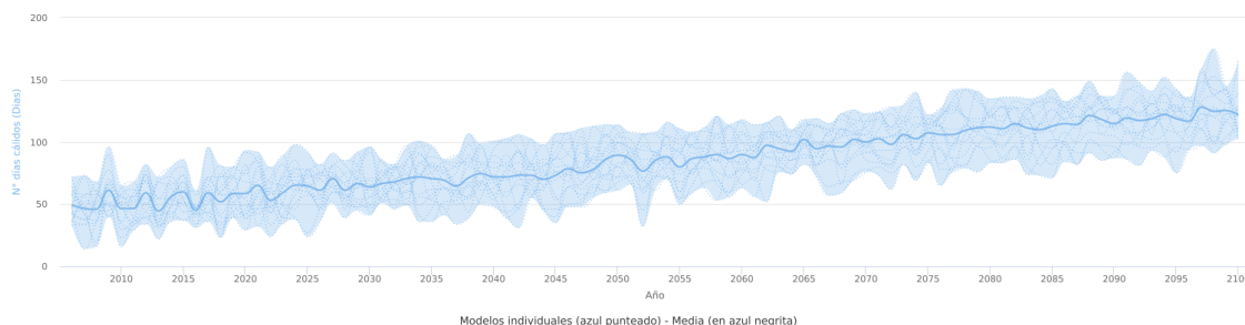
Escenarios AdapteCCa - N° días cálidos - Datos en rejilla ajustados (media) - RCP 8.5 - Año completo - Borriana/Burriana (Comunitat Valenciana)
