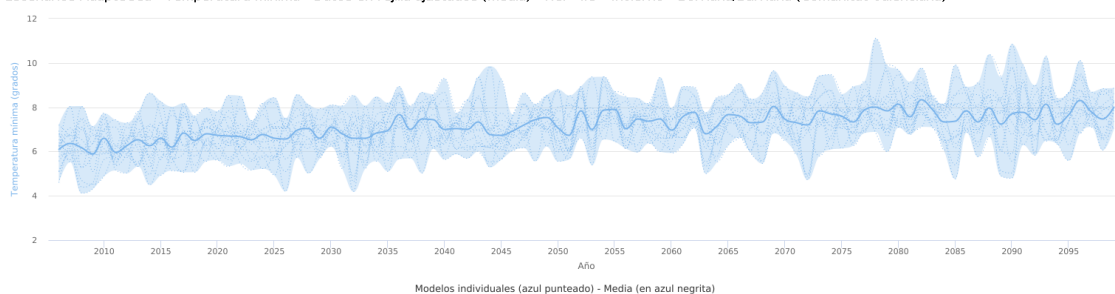
Escenarios AdapteCCa - Temperatura mínima - Datos en rejilla ajustados (media) - RCP 4.5 - Invierno - Borriana/Burriana (Comunitat Valenciana)
