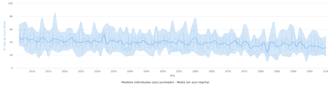
Escenarios AdapteCCa - N° días de lluvia - Datos en rejilla ajustados (media) - RCP 8.5 - Año completo - Burriana/Burriana (Comunitat Valenciana)
