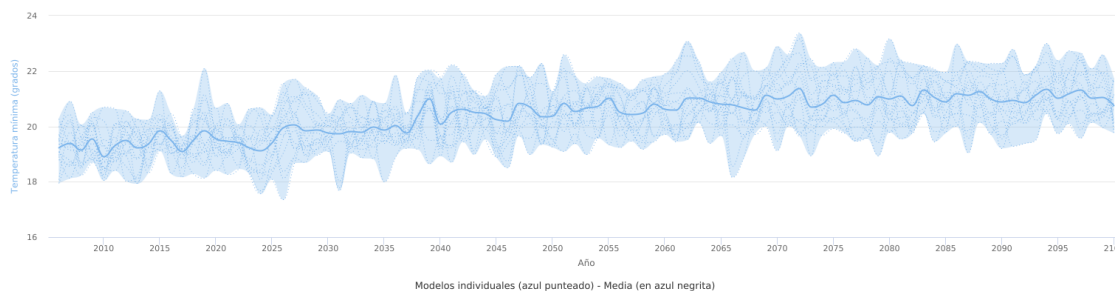
Escenarios AdapteCCa - Temperatura mínima - Datos en rejilla ajustados (media) - RCP 4.5 - Verano - Borriana/Burriana (Comunitat Valenciana)
