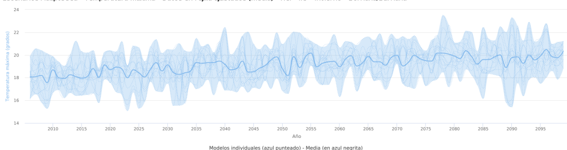
Escenarios AdapteCCa - Temperatura máxima - Datos en rejilla ajustados (media) - RCP 4.5 - Invierno - Borriana/Burriana
