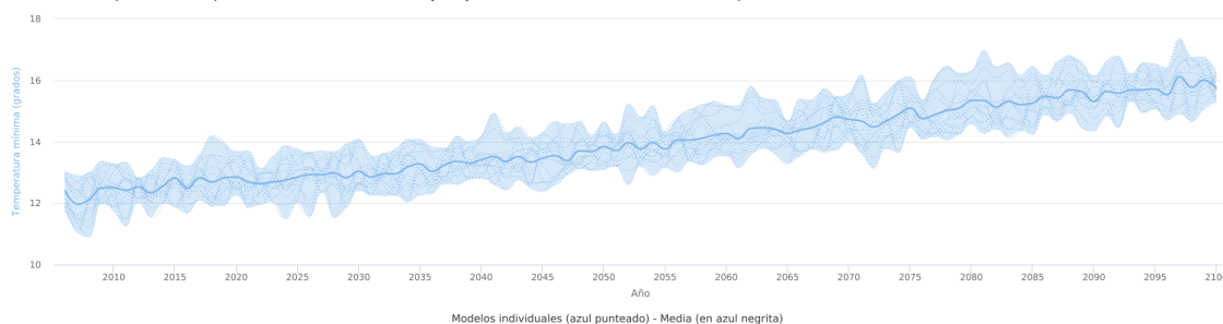
Escenarios AdapteCCa - Temperatura mínima - Datos en rejilla ajustados (media) - RCP 8.5 - Año completo - Borriana/Burriana (Comunitat Valenciana)
