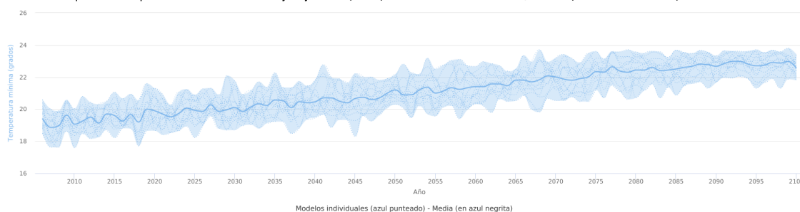
Escenarios AdapteCCa - Temperatura mínima - Datos en rejilla ajustados (media) - RCP 8.5 - Verano - Borriana/Burriana (Comunitat Valenciana)
