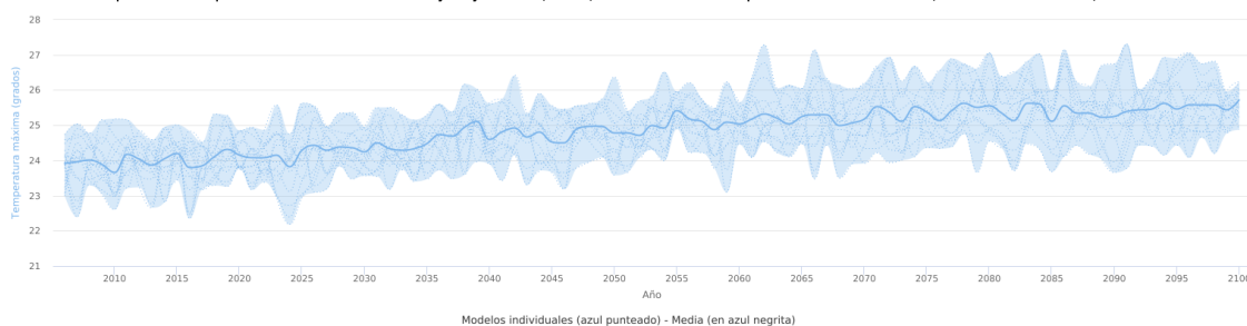
Escenarios AdapteCCa - Temperatura máxima - Datos en rejilla ajustados (media) - RCP 4.5 - Año completo - Borriana/Burriana (Comunitat Valenciana)
