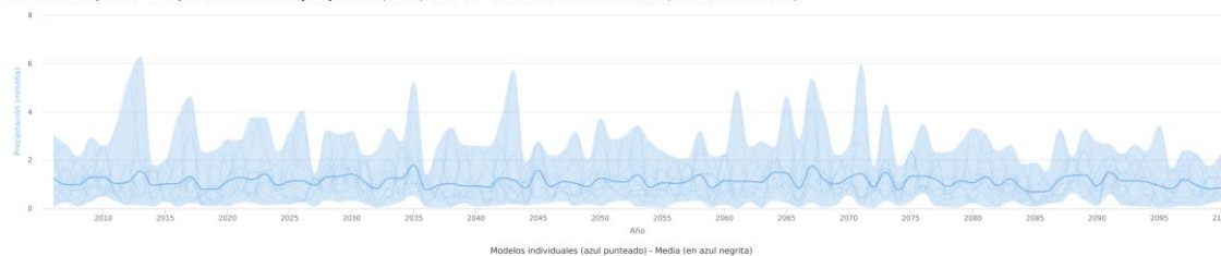
Escenarios AdapteCCa - Precipitación - Datos en rejilla ajustados (media) - RCP 4.5 - Primavera - Borriana/Burriana (Comunitat Valenciana)
