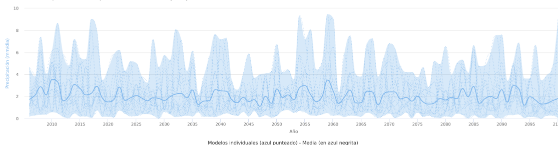
Escenarios AdapteCCa - Precipitación - Datos en rejilla ajustados (media) - RCP 8.5 - Otoño - Borriana/Burriana (Comunitat Valenciana)
