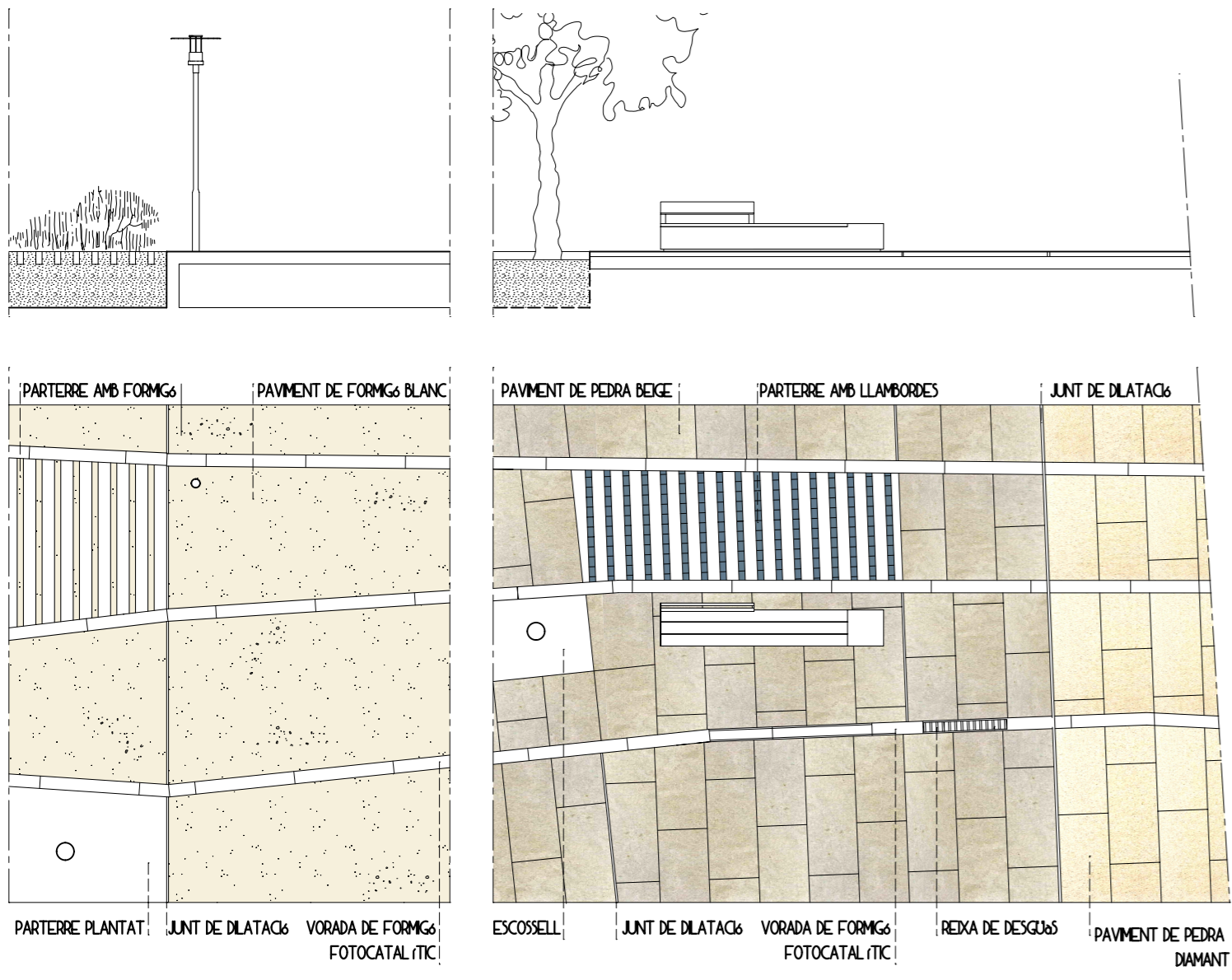
PAVIMENTS E: 1/100 ESCALA GRÀFICA 1/100
