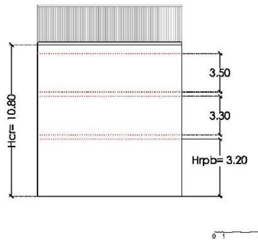
FACHADA PROTEGIDA
