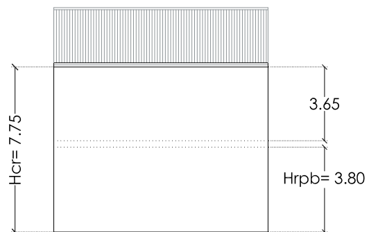
Esquema de Fachada
