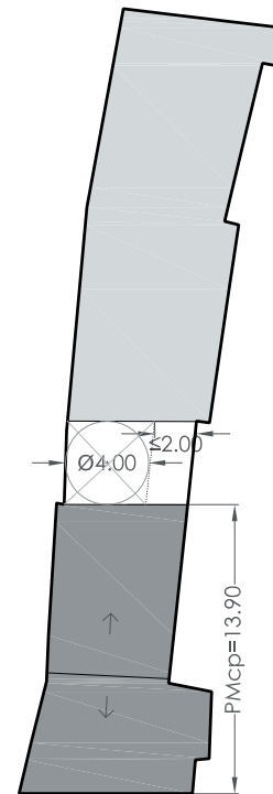
Esquema de ocupación - Planta- E: 1/400
