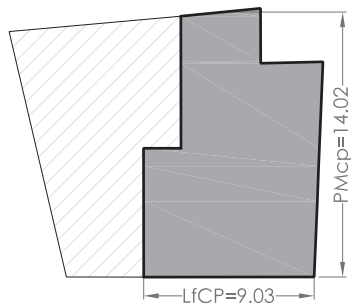
Cuerpo principal protegido E: 1/400
