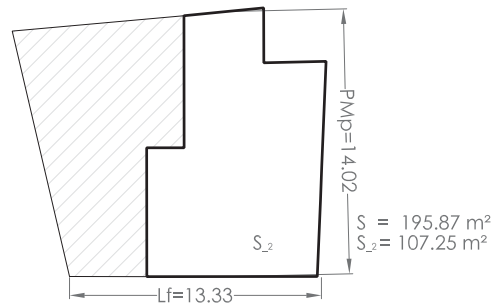
Planta E: 1/400
