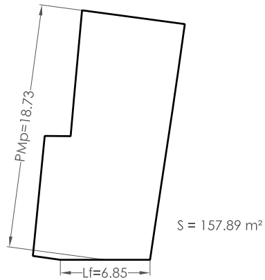
Planta E: 1/400
